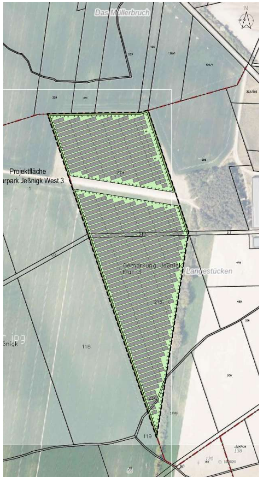
Abbildung 2: Belegungsplan der PVA - Quelle: Auftraggeber
