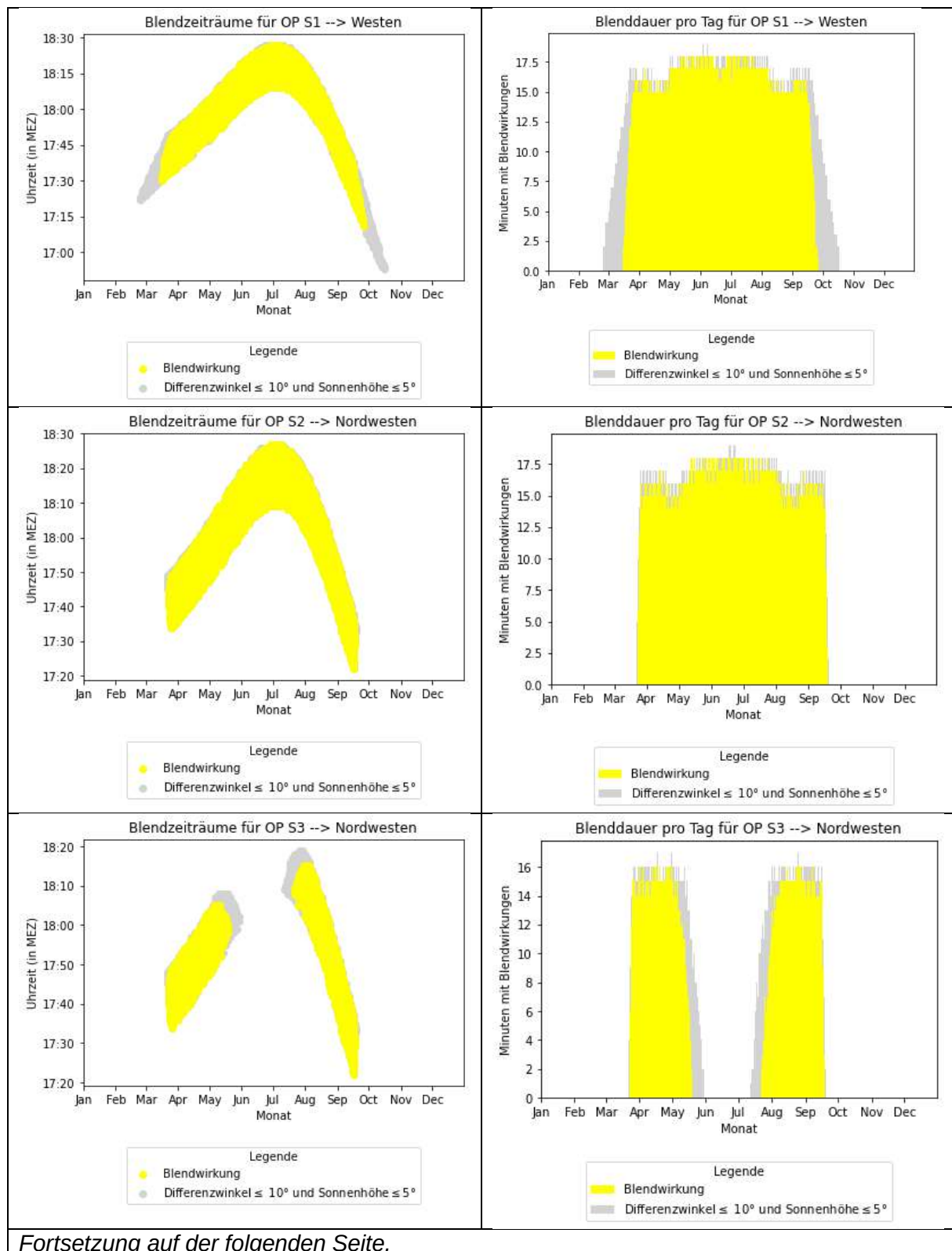
Ergebnisdiagramme 1: Reflexionen in das erhebliche Sichtfeld von Fahrzeugführern (Hindernisse nicht berücksichtigt)
