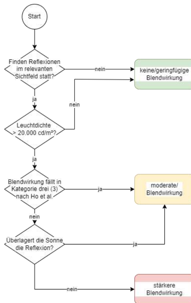
Abbildung 17: Bewertungsmethodik als Entscheidungsbaum für PVA-bedingte Blendwirkungen auf Piloten während eines Landeanflugs oder beim Rollen am Boden
