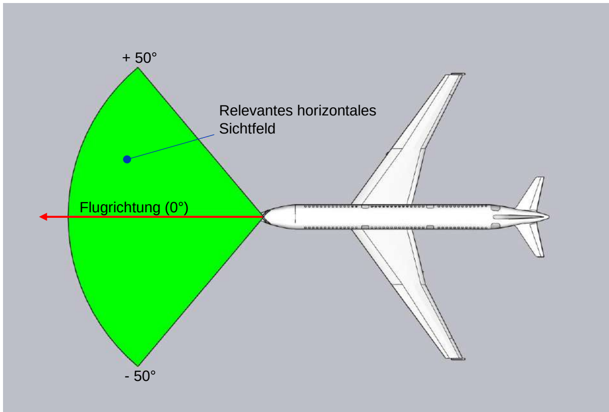
Abbildung 14: Darstellung des relevanten horizontalen Sichtfelds: Außerhalb von 50° zur Flugrichtung sind Reflexionen irrelevant. - Quelle Abbildung: Eigene Abbildung
