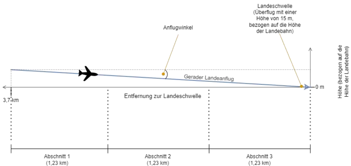
Abbildung 16: Skizze eines modellierten/simulierten Anflugs
