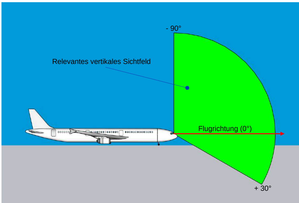
Abbildung 15: Darstellung des relevanten vertikalen Sichtfelds: Ab 30° gegen Boden ist dieses eingeschränkt. - Quelle Abbildung: Eigene Abbildung
