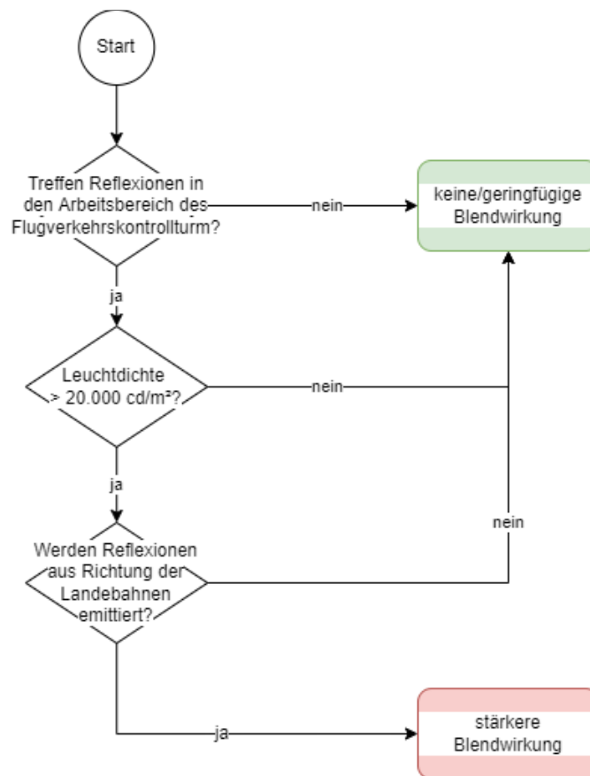
Abbildung 18: Bewertungsmethodik als Entscheidungsbaum für PVA-bedingte Blendwirkungen auf Fluglotsen im Flugverkehrskontrollturm
