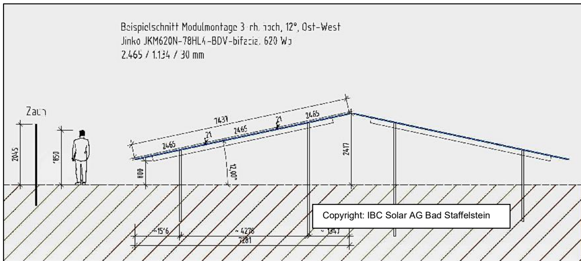
Abb. 20: Prinzipskizze der Modultische in Nord-Süd-Reihung bei Verwendung von bifazialen PV-Modulen. Hierbei sind die Modulflächen in Ost-West-Richtung ausgerichtet.
