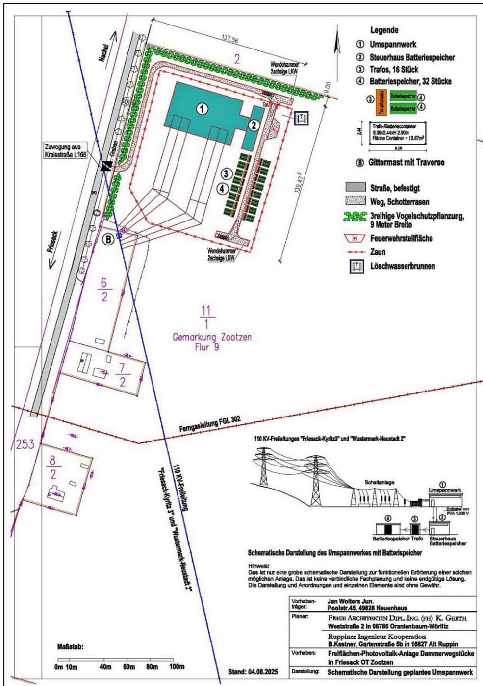
Abb. 30: Die funktionale Einheit des Netzverknüpfungspunktes mit den beiden neuen Umspannwerken und den integrierten Batteriespeichern. (Zeichng.: RIK-Kathleen Gerth)
