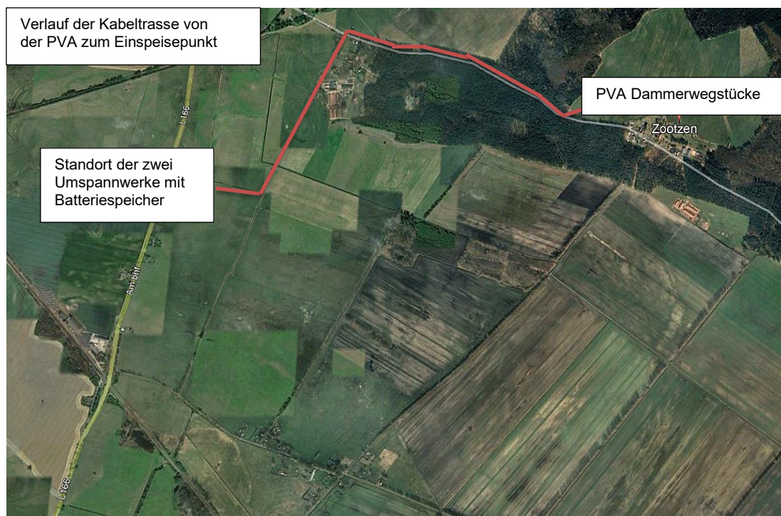
Abb. 29: Ungefährer Trassenverlauf des einspeisenden Erdkabels von der PVA zum Einspeisepunkt an der Landstraße L 166, Nähe Bahnhof Friesack. Die Entfernung beträgt ca. 3 km. (Quelle: Google)
