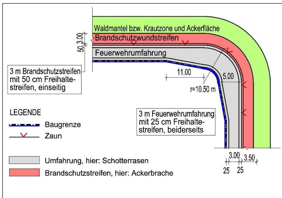
Abb. 23: Prinzipbild der Umfahrung um die PV-Anlage mit schematischer Darstellung der Kurvenausführung des extensiven Wiesenstreifens, der zur Umfahrung der künftigen Photovoltaikfelder von jeglicher Bebauung und Bepflanzung freizuhalten ist. (Zeichng. RIK: Kathleen Gerth)
