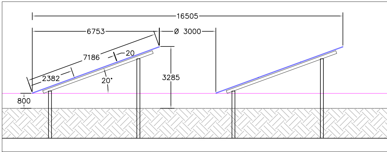
exemplarische Seitenansicht (alle Maße in Millimeter)
