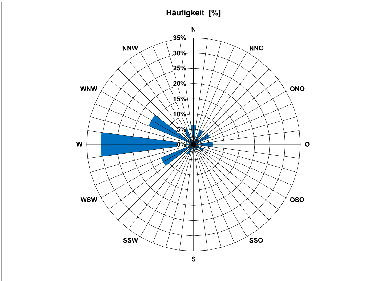
Abbildung 2: Windrose der gefilterten Daten in 200 m Höhe nach Szenario 2 für die Jahre 1999 bis einschließlich 2023 am Standort Wulkow Erweiterung 1
