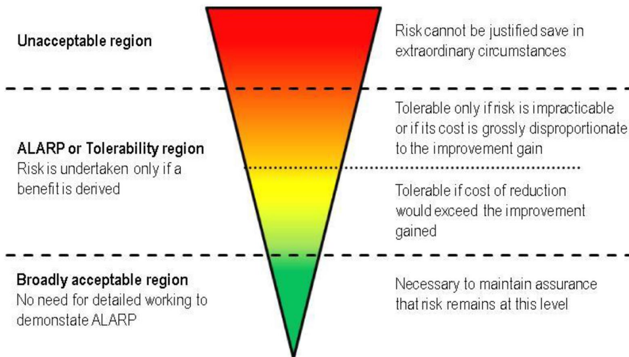
Abbildung 6: ALARP-Prinzip [7]
