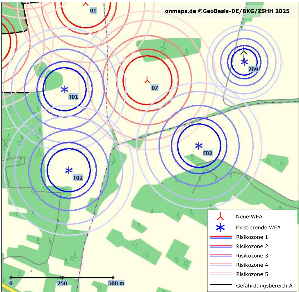
Abbildung 5: WEA 07 ohne Gefährdungsbereich
