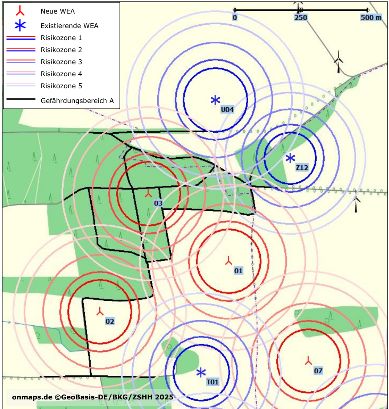
Abbildung 4: WEA 01 bis 03 mit GB A
