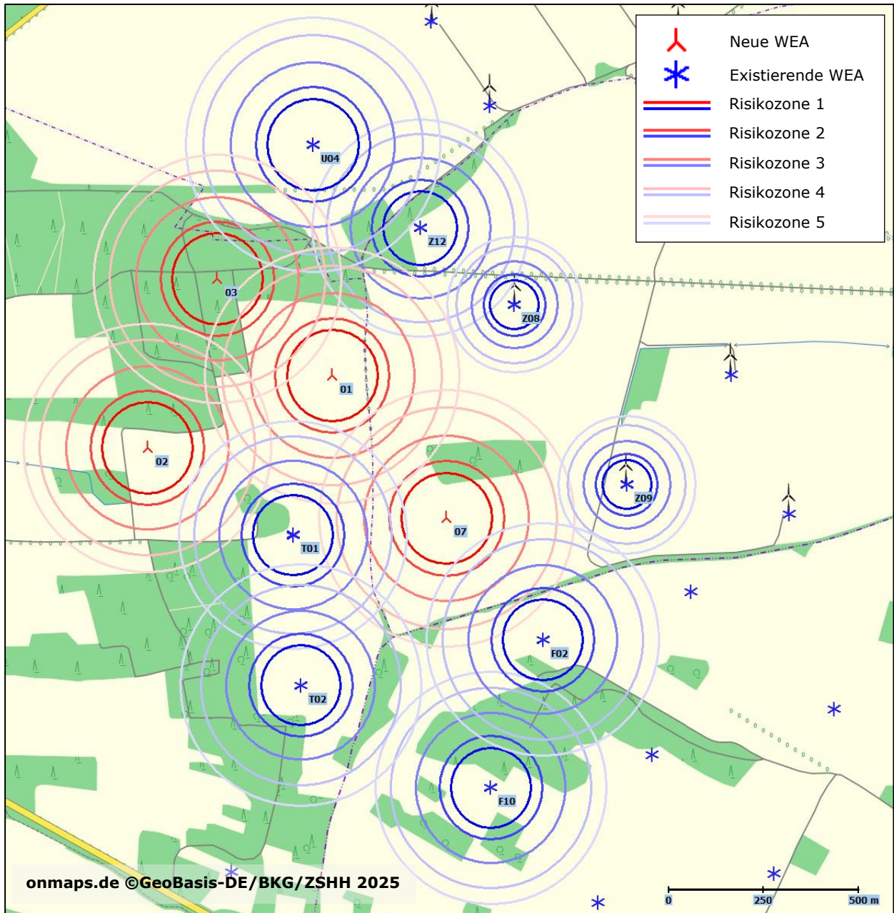
Abbildung 3: Risikozonen
