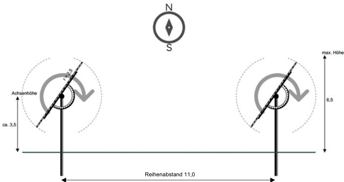
Abbildung 19 Prinzipskizze Anlagenlayout, Werte gerundet in Metern (Quelle: Elysium Solar Schenkendorf GmbH)
