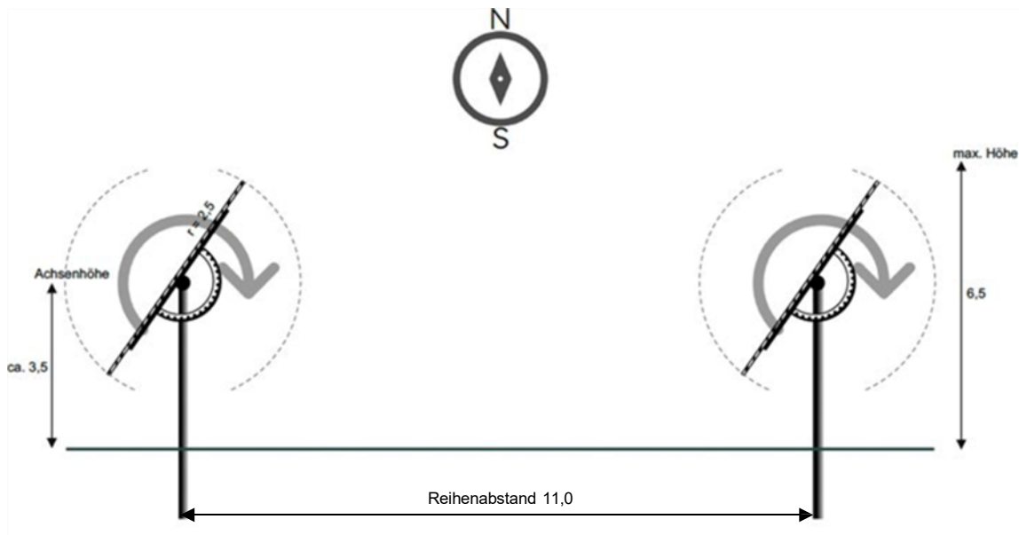
Abbildung 2: Darstellung Agri-PV-Anlage
