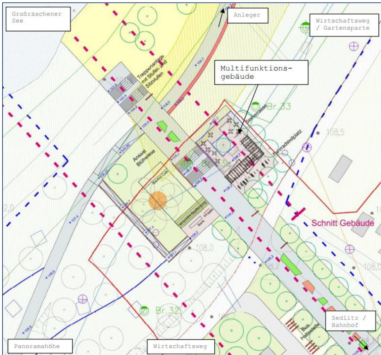
Abbildung 2: Auszug vom Konzept zur Gestaltung des Ostufers des Großräschener Sees (Quelle: pahn Ingenieure)
