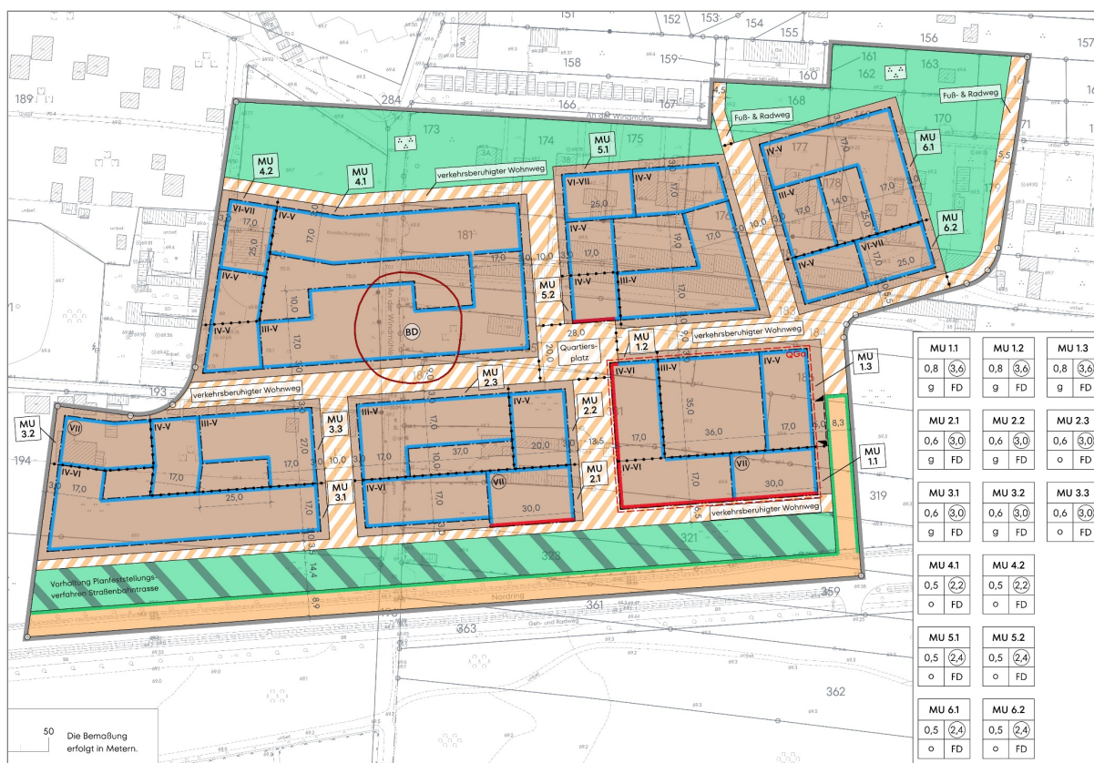
Abbildung 2.2: B-Plan Vorentwurf (MAYERWITTIG 2026, o. M.)
