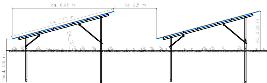
Abbildung 3: Schnittzeichnung - Quelle: Auftraggeber
