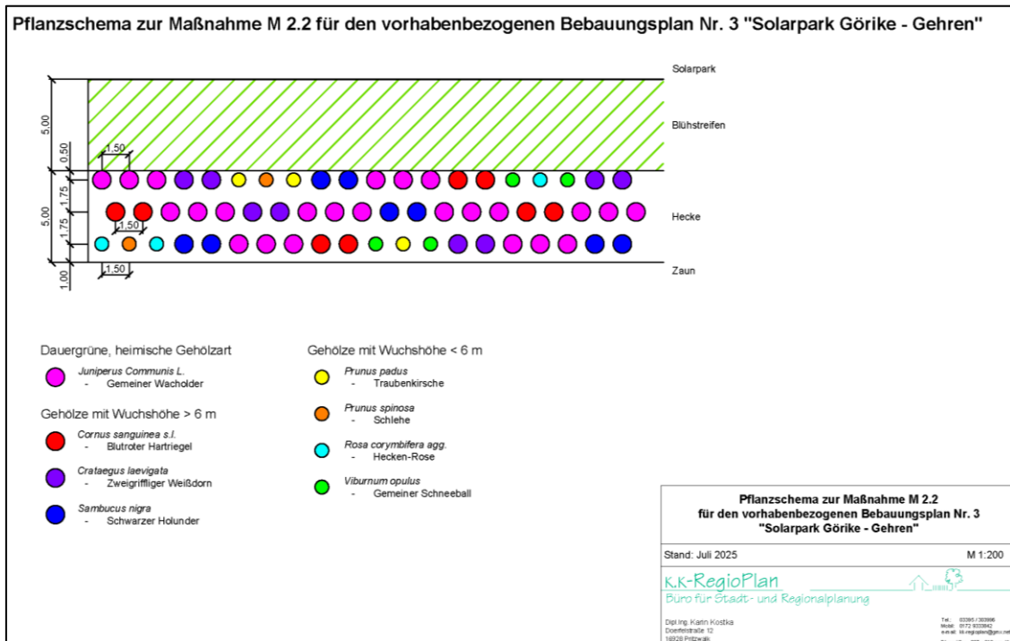
Abbildung 13 Pflanzschema für die Maßnahme M2.2
