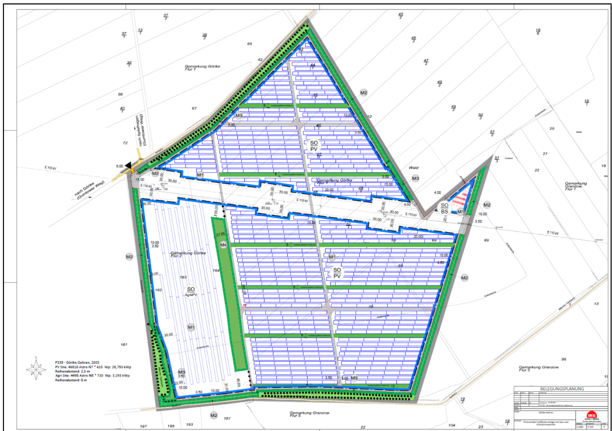
Abbildung 14 Vorläufiger Modulbelegungsplan „Solarpark Görike- Gehren“, Stand 01.08.2025
