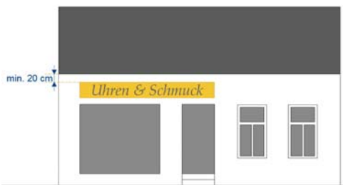
Bei eingeschossigen Gebäuden müssen Werbeanlagen einen Mindestabstand von 20 cm zur Traufe einhalten
