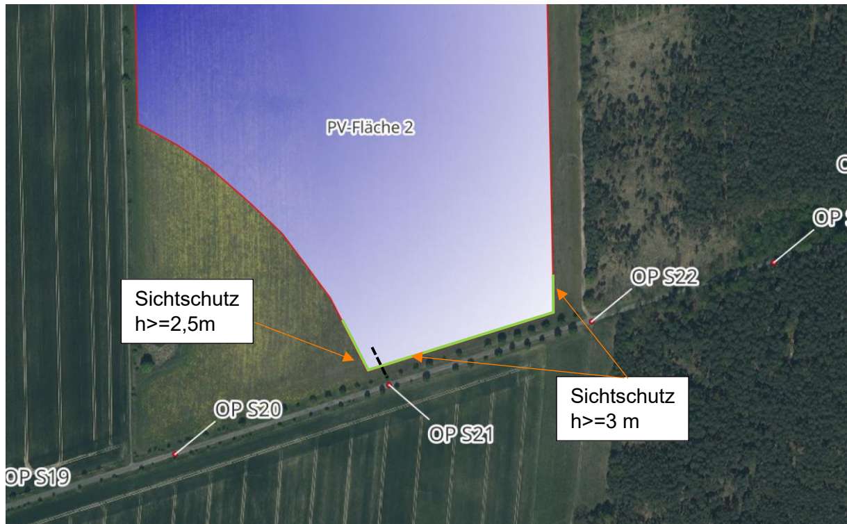
Abbildung 13: Positionen und Höhen des Sichtschutzes bei PV-Fläche 2
