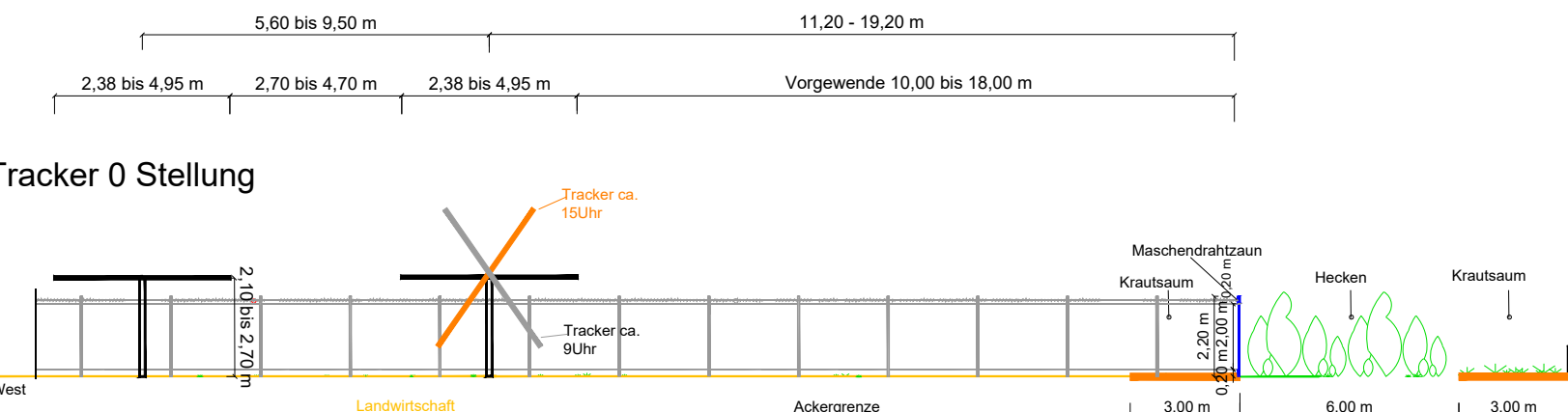
Standardschnitt Flächen C-D-E
