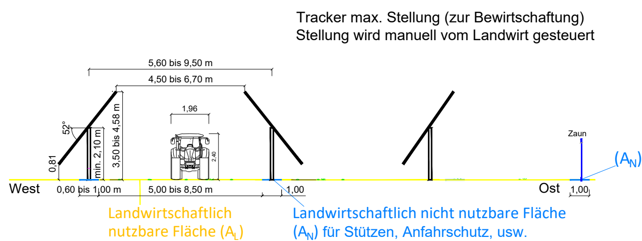
Schnitt Bewirtschaftung Flächen C-D-E
