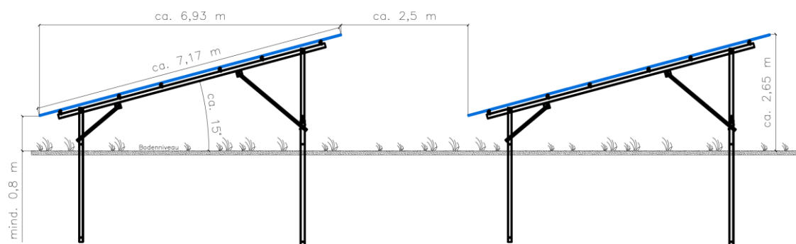
Abbildung 3: Schnittzeichnung - Quelle: Auftraggeber
